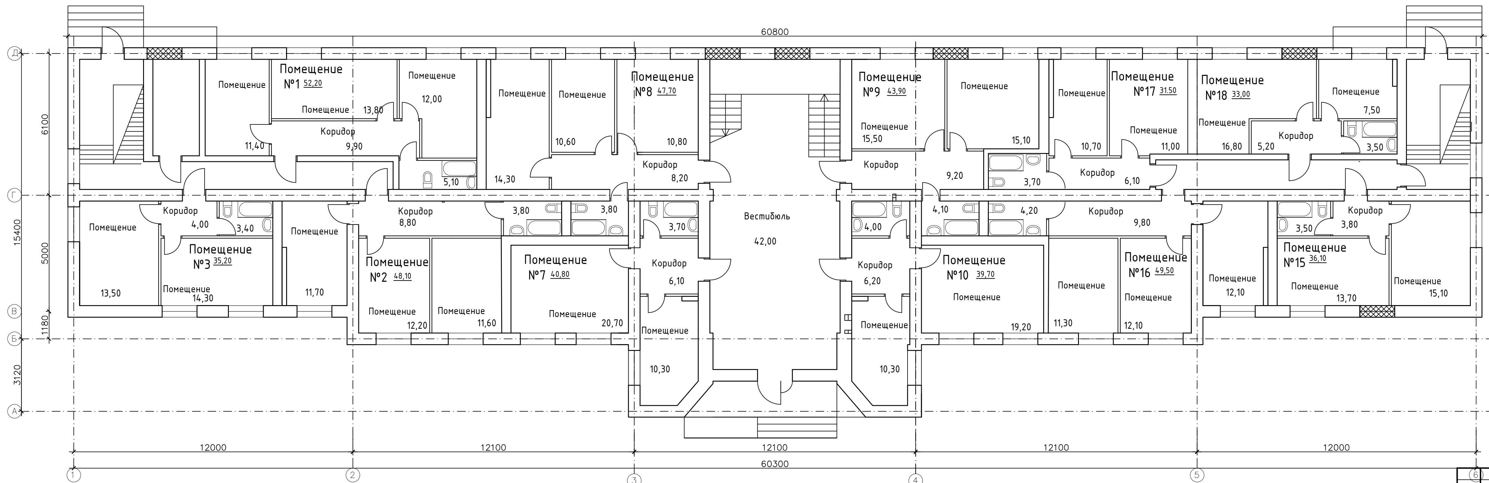
План 1-го этажа на отм. 0.000.
